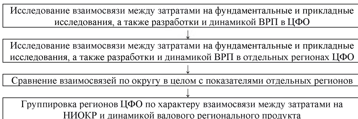
Рисунок 1 – Этапы оценки взаимосвязи между затратами на научно-инновационное развитие и величиной ВРП
